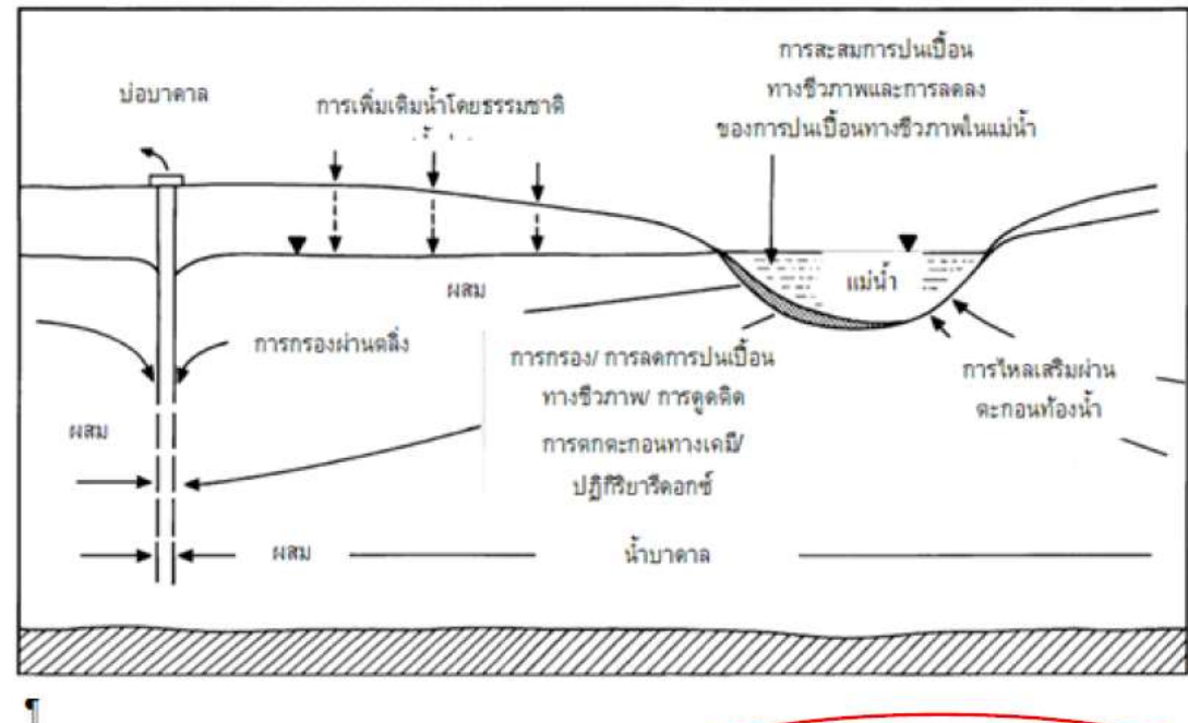
ภาพที่ 3 → ลักษณะของการพัฒนาแหล่งน้ำระบบ RBF (Hiscock & Grischek, 2002)
