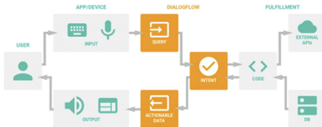
รูปที่ 3.1 รูปแสดงการทำงานของDialogFlow
